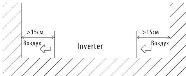
Рисунок 7.1: Пример установки
